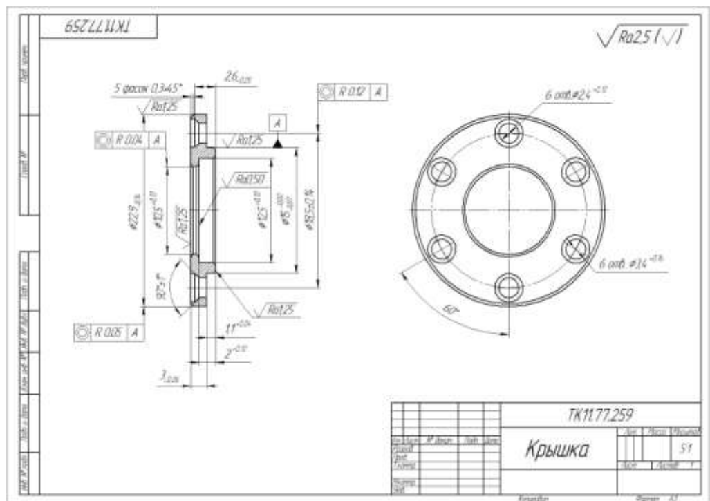
Рисунок 6 – Чертеж детали
