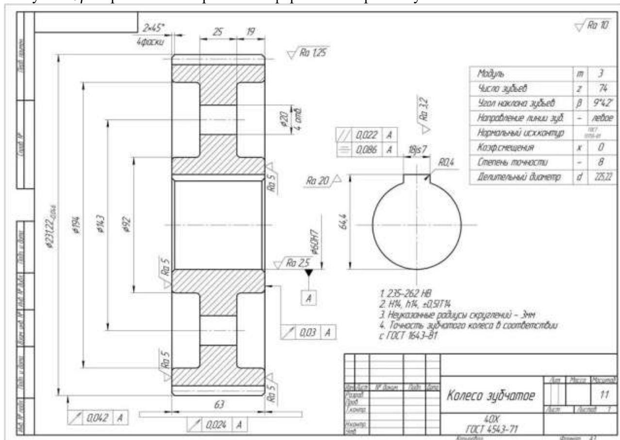
Рисунок 5 –Зубчатое колесо
