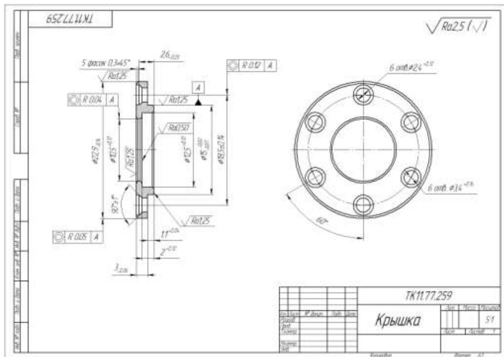
Рисунок 6 – Чертеж детали
